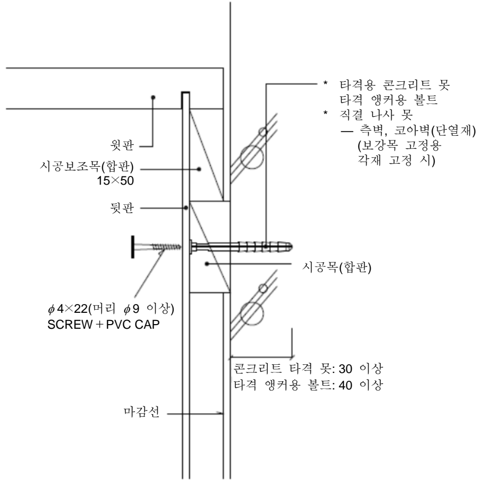
그림 1 — 시공목 고정
